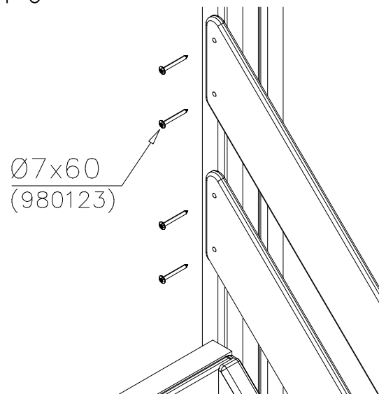
DET 6
