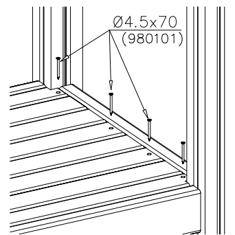
DET 3
