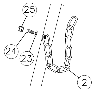
DET 6
